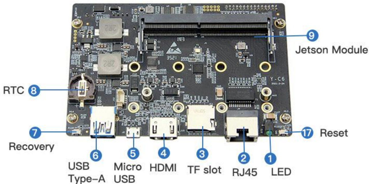
Y-C6载板正面接口指示图
