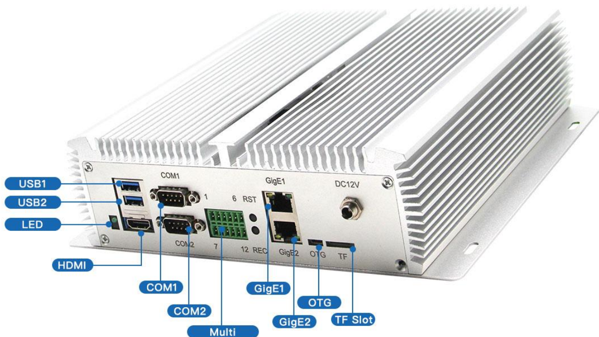
8F5E2 正面接口标识图
