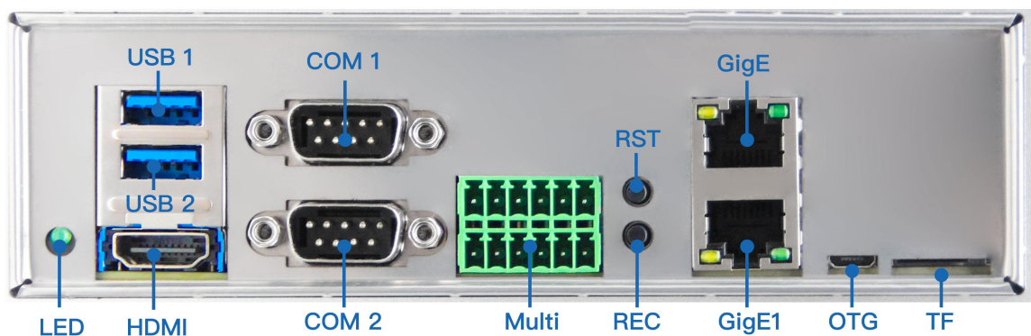
8F1E1 接口指示图
